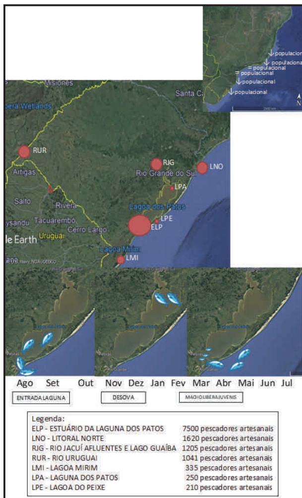
Figura 2: Representação esquemática da condição da população de bagre no sul e sudeste do Brasil, número de pescadores artesanais no Rio Grande do Sul e ciclo biológico da espécie
